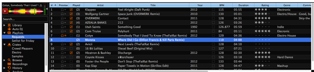
Figure 1: Mixxx knjižnica
