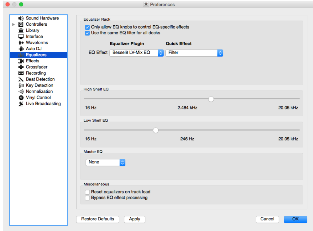
Figure4: Nastavitve izravnalnika
